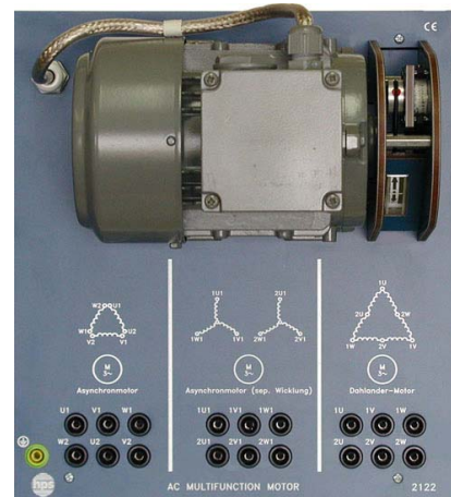
AC MULTIFUNCTION MOTOR (Typ 2122)
